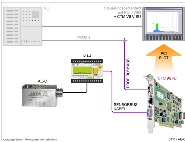
Anwendungsbeispiel: AE-C mit KU-4 im CTM Werkzeug- und Prozessüberwachungssystem
