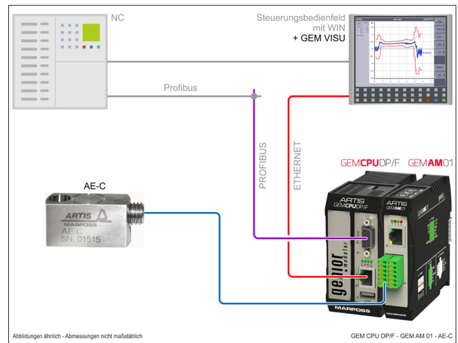
Anwendungsbeispiel: AE-C mit AM-01 im GENIOR MODULAR Werkzeug- und Prozessüberwachungssystem
